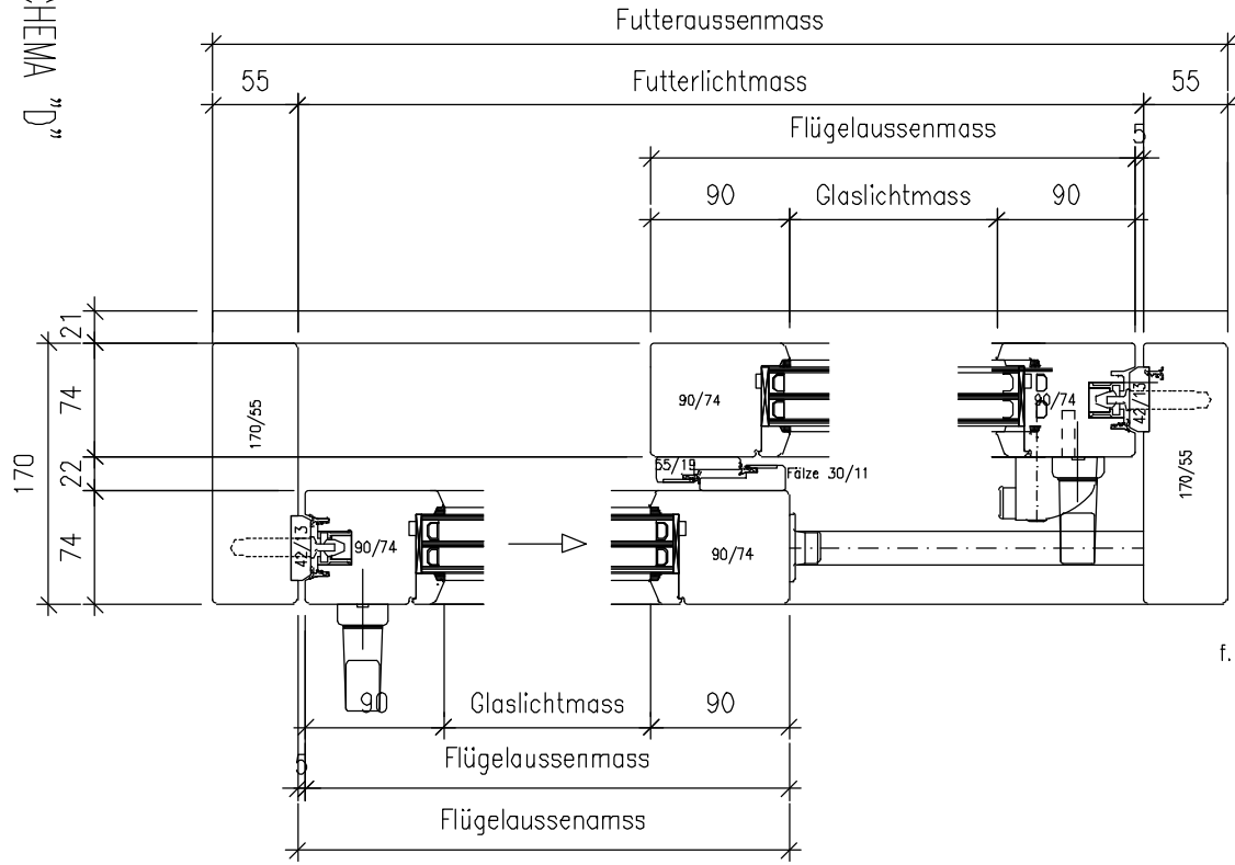
GRUNDRISS
