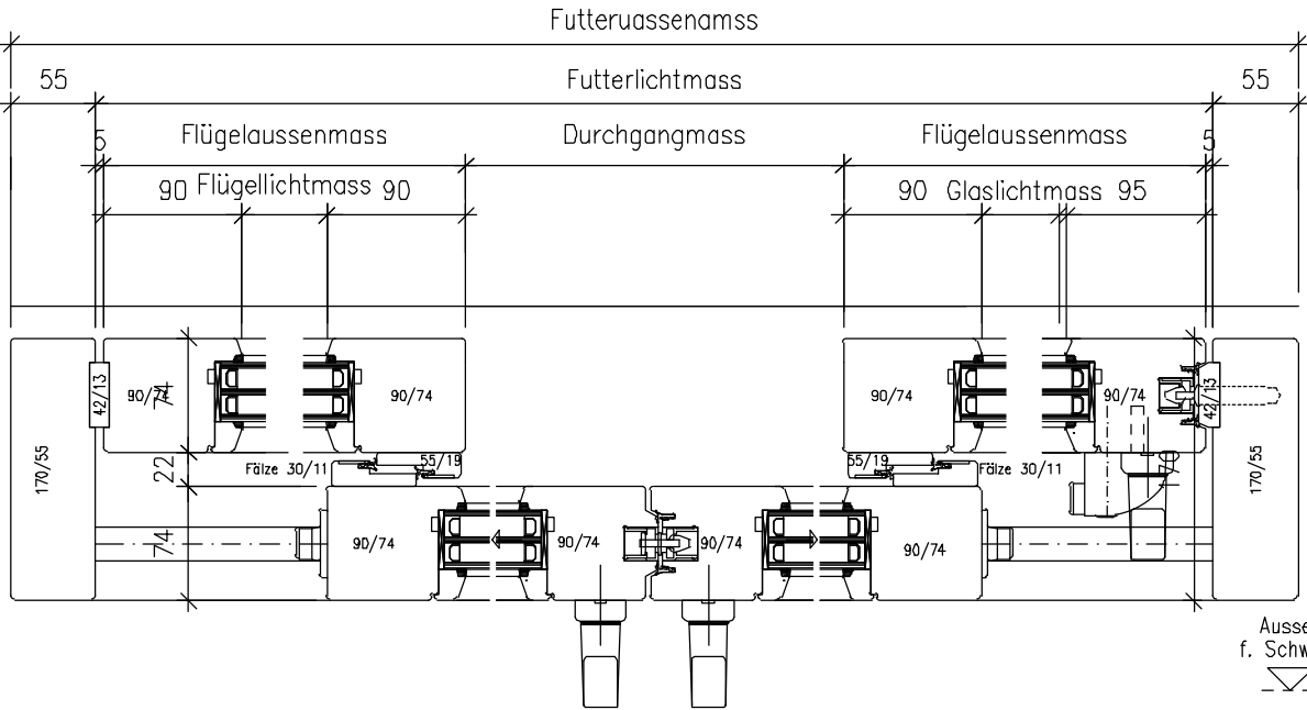
GRUNDRISS
