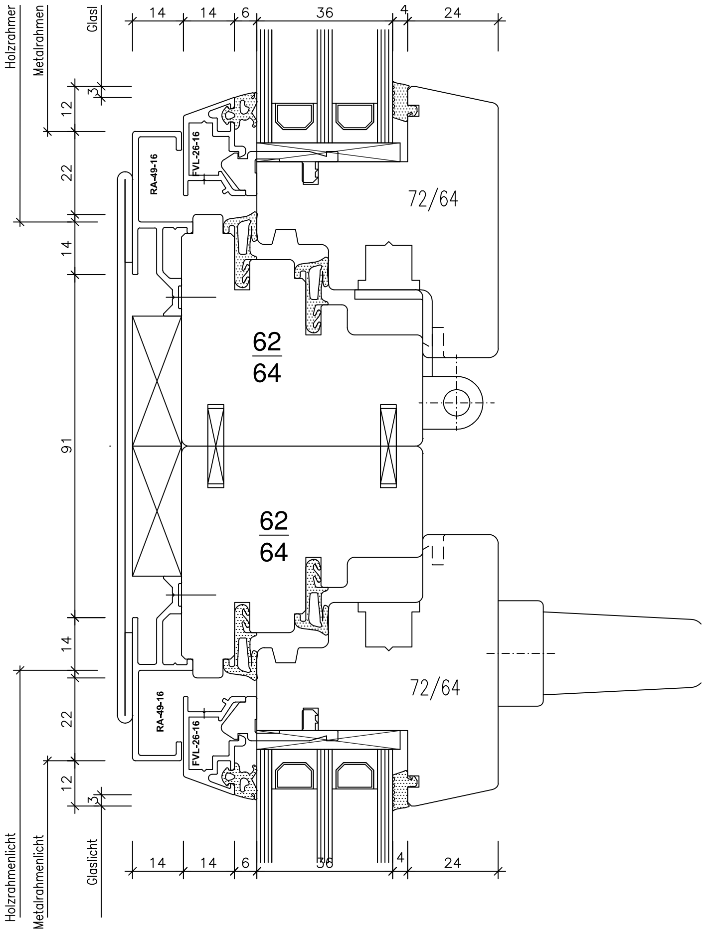
Fenster Sirius D 64/64 Setzholz Rahmenezusammenbau "Standart" 4,03
