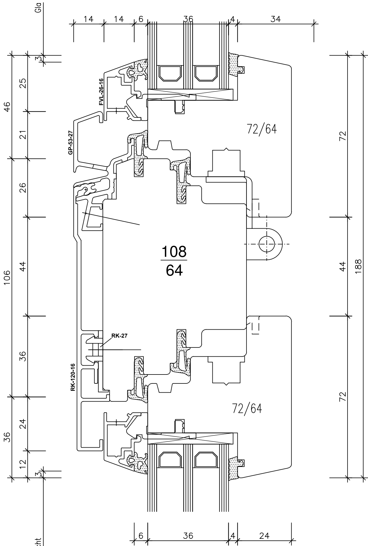
Fenster Sirius D 64/64
