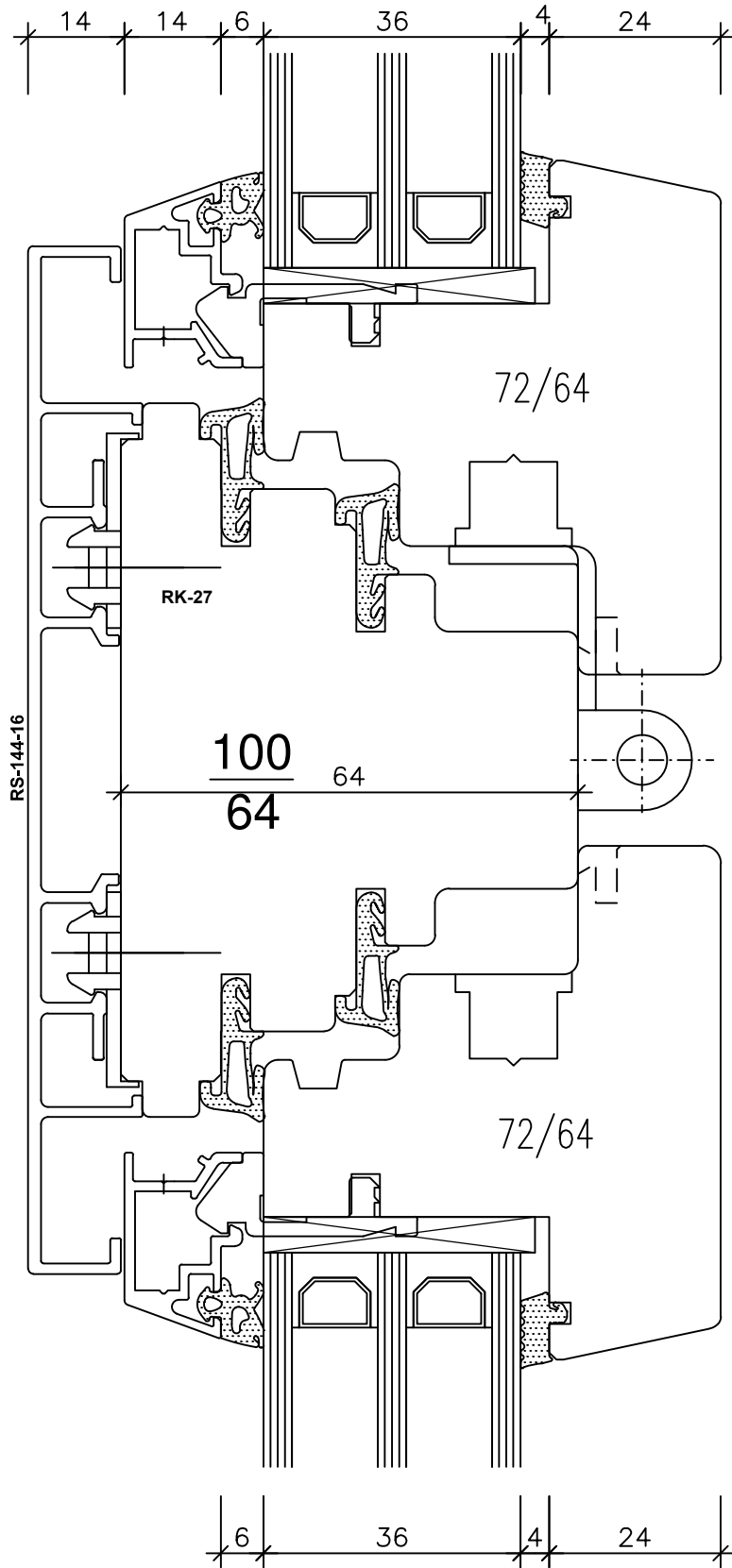
Setzholz "Standart" 4,01
