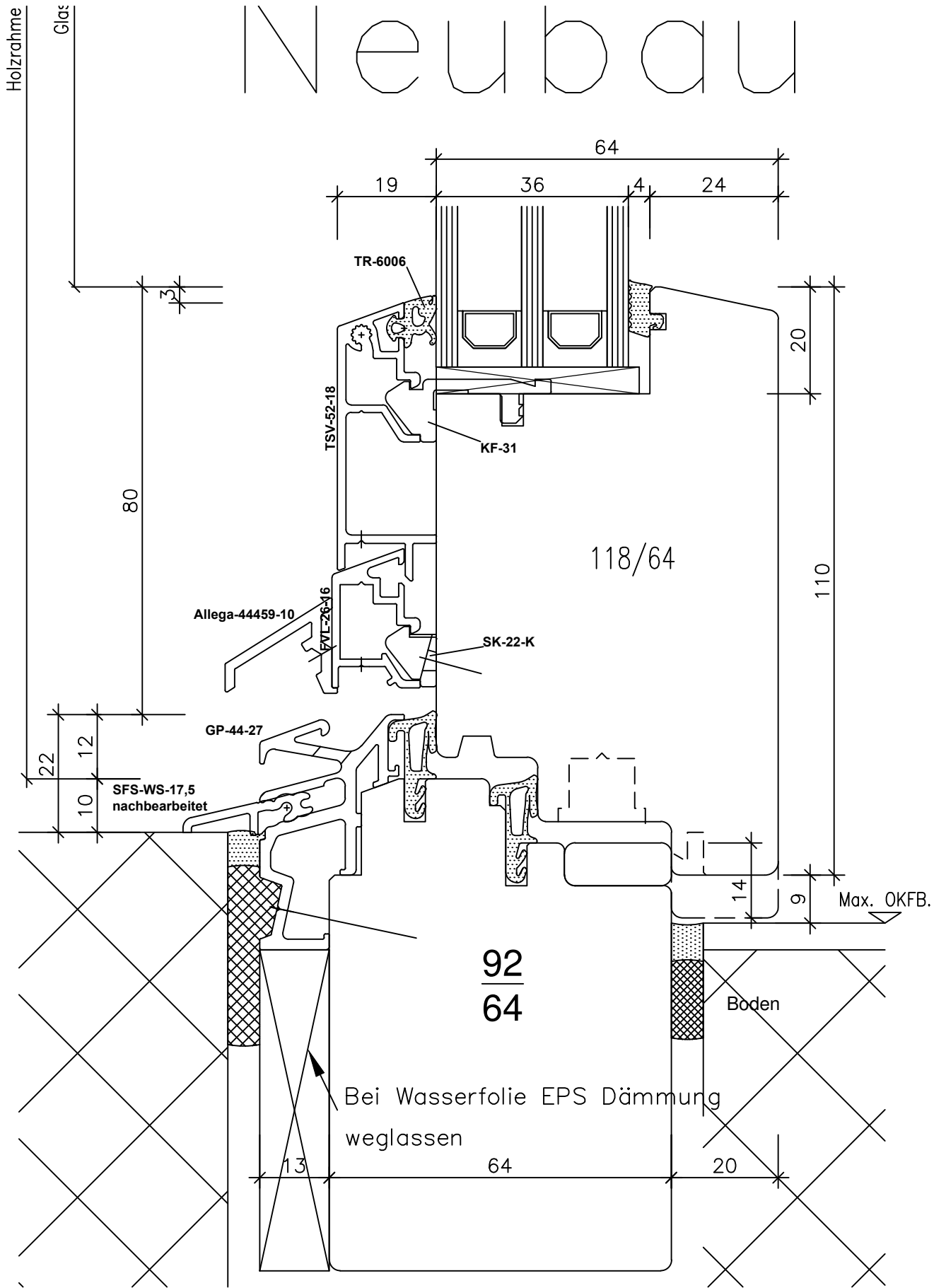
Fenster Sirius D 64/64
