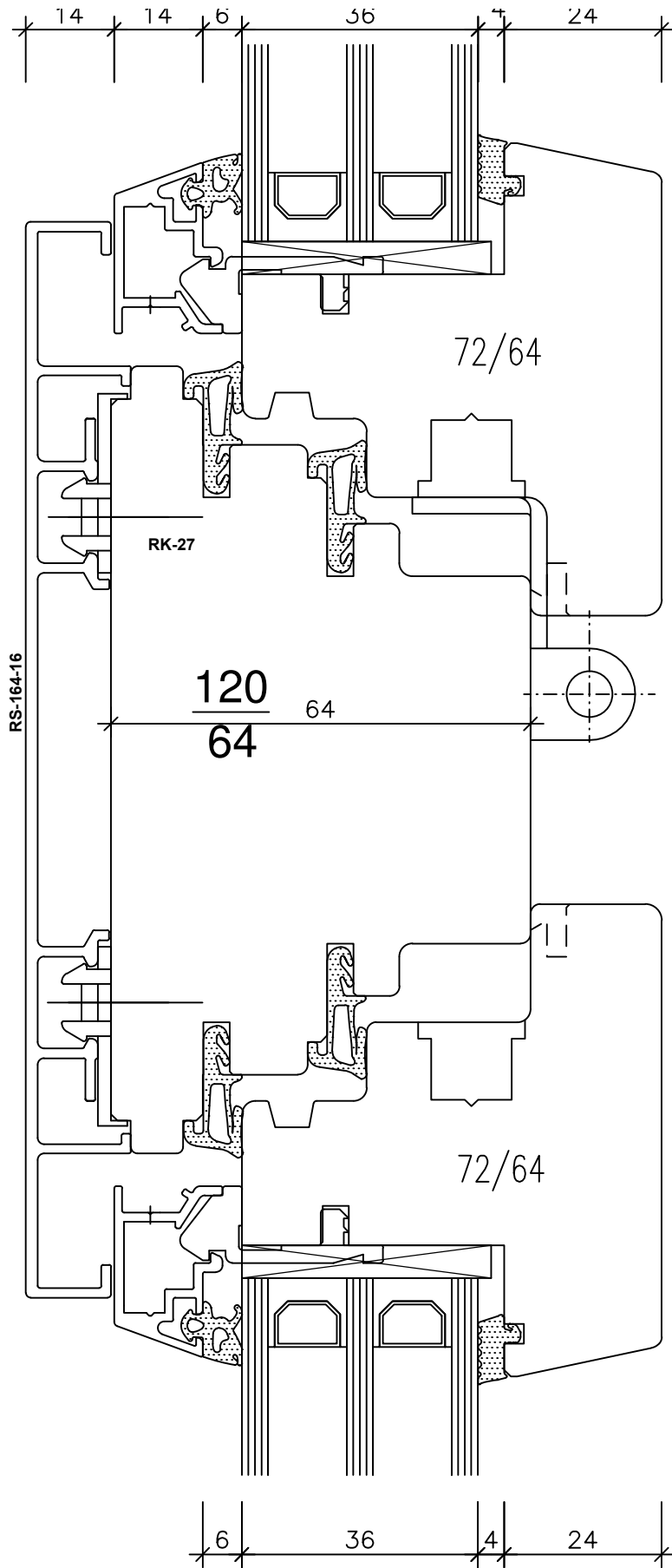
Setzholz "Standart" 4,02
