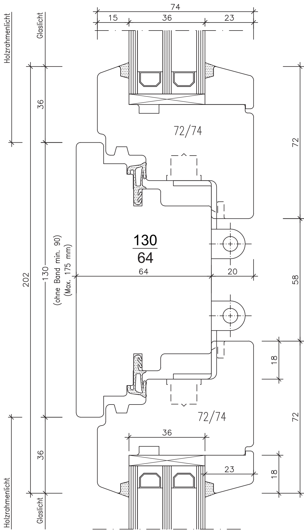
Fenster Sirius H 64/74
