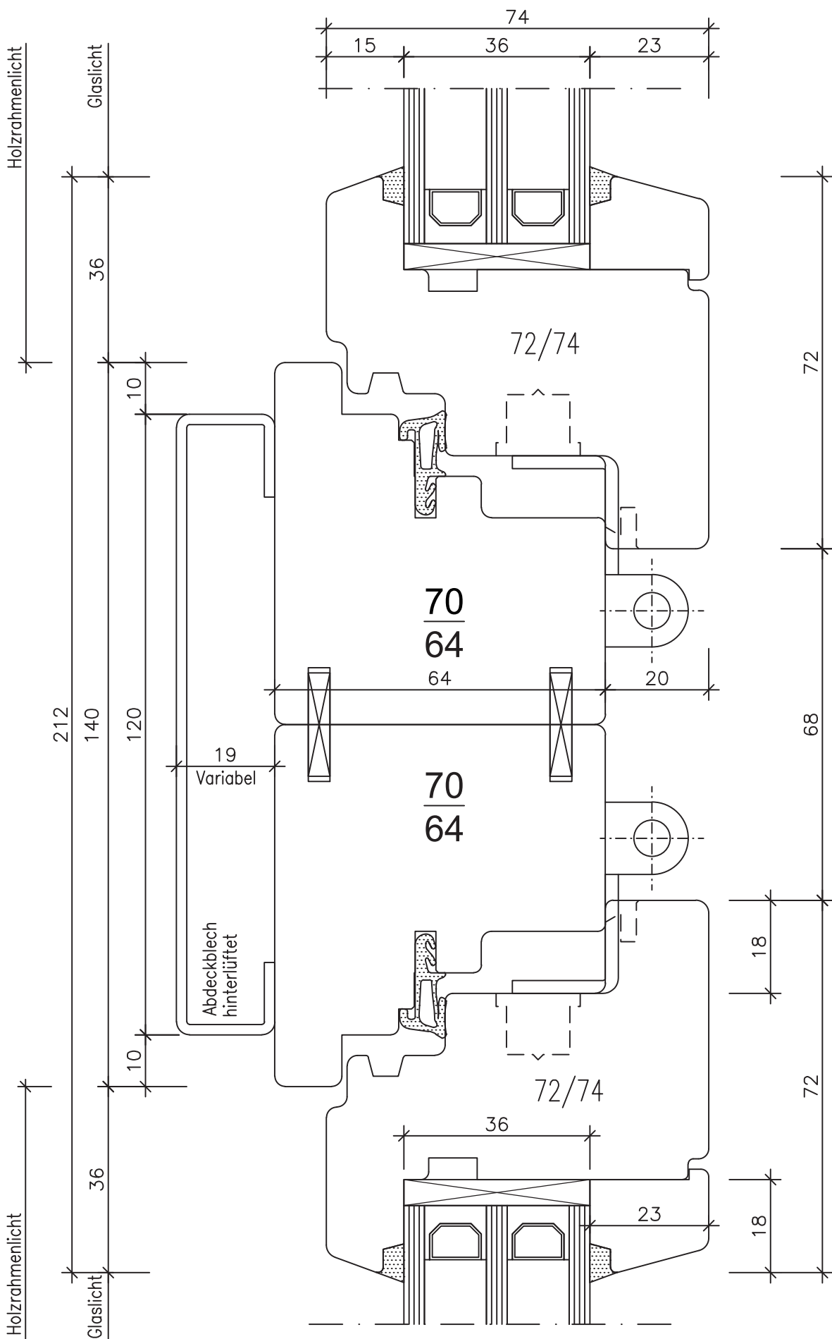
Fenster Sirius H 64/74
